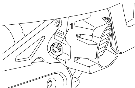
1. Öleinfüllöffnung
