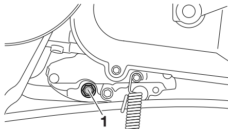
1. Motoröl-Ablassschraube A
