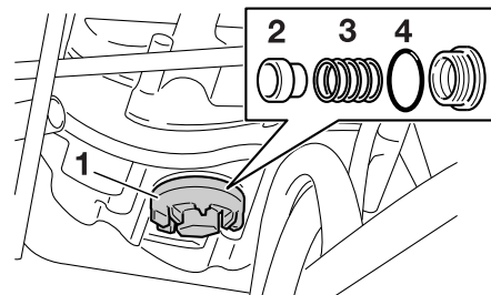
1. Cavilha de drenagem do óleo do motor B 2. Coador 3. Mola de compressão 4. Anel de vedação em O
