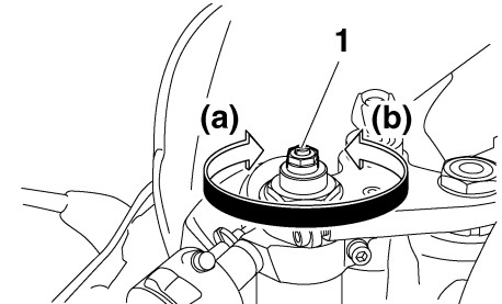
1. Parafuso ajustador da força amortecedora de recuo
