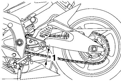
1. Antriebsketten-Durchhang
