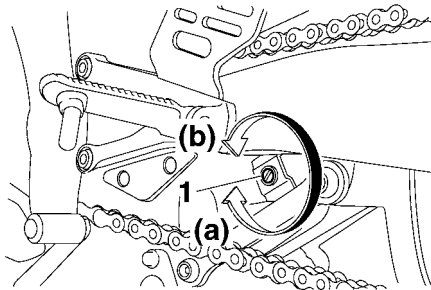
1. Zugstufendämpfungs-Einstellschraube
