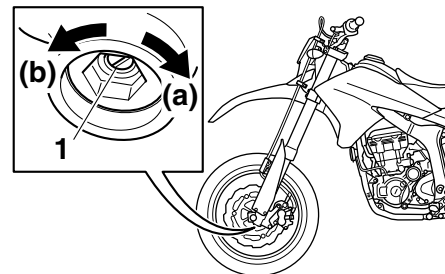
1. Stelschroef voor inveerdemping
