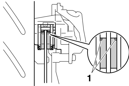
1. Verschleißanzeiger
