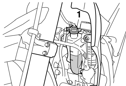
1. Kühlflüssigkeits-Ausgleichsbehälterdeckel
