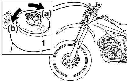
1. Zugstufendämpfungs-Einstellschraube
