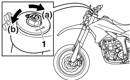
1. Zugstufendämpfungs-Einstellschraube
