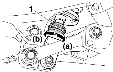
1. Quadrante di regolazione dello smorzamento in estensione
