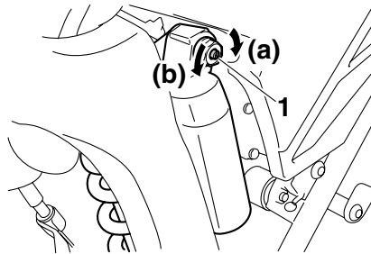
1. Vite di regolazione dello smorzamento in compressione
