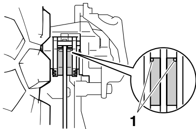
1. Indicador de desgaste
