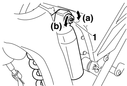
1. Parafuso ajustador da força amortecedora de compressão
