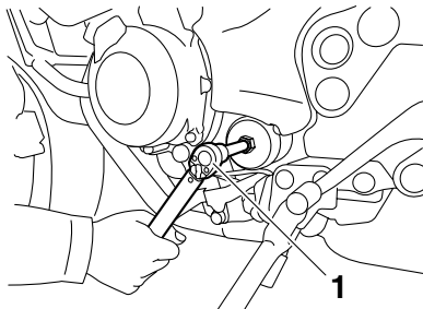
1. Clé dynamométrique
