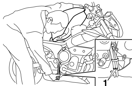
1. Ausgangsstellung (Farbmarkierung)
