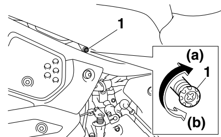
1. Leerlauf­einstellschraube
