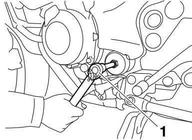
1. Momentnyckel
