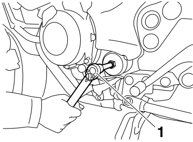
1. Chave de binário
