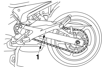
1. Folga da corrente de transmissão
