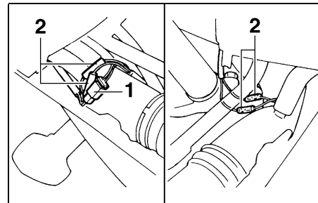
1. Fiche rapide de veilleuse 2. Connecteur de clignotant (× 2)
