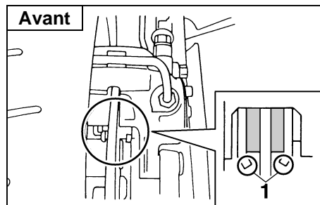
1. Rainure d'indication d'usure de plaquette de frein (× 2)
