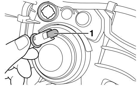
1. Standlichtlampe
