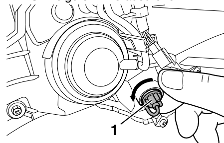
1. Blinkerlampefassung
