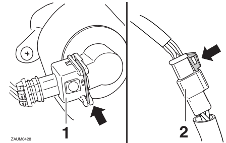
1. Blinkerkabel-Steckverbinder
