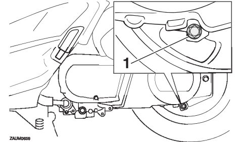
1. Achsgetriebeöl-Ablassschraube
