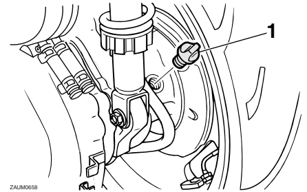
1. Achsgetriebeöl-Einfüllschraubverschluss
