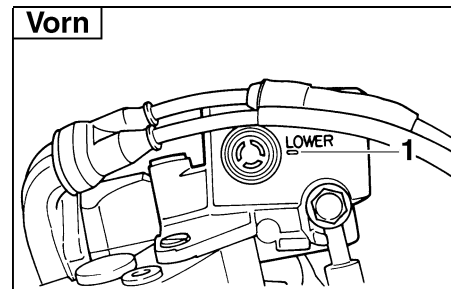
1. Minimalstand
