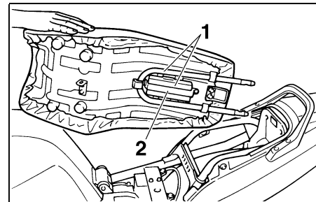
1. Bügelschloß 2. Befestigungsgummi
