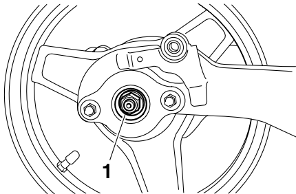
1. Écrou d'axe
