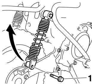
1. Vis de montage d'amortisseur arrière
