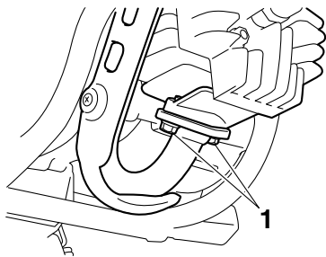
1. Vis de tubulure d'échappement
