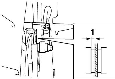
1. Remvoeringdikte
