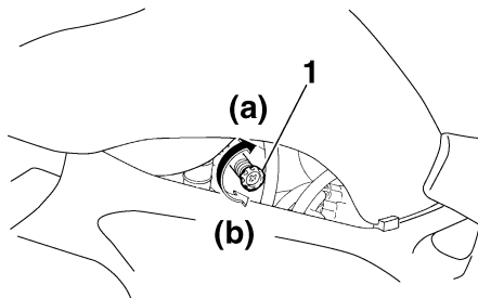
1. Tornillo de ajuste del ralenti
