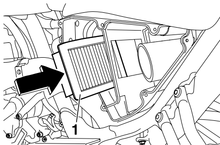
1. Elemento filtrante
