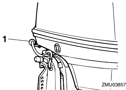
1. Εξάρτημα πλυσίματος
