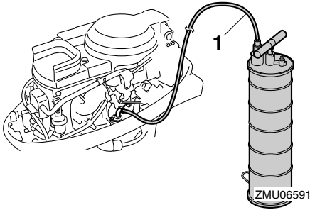
1. Ölwechsler
