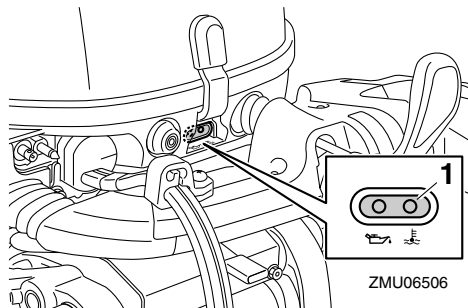
1. Warnanzeige
