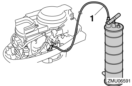
1. Vidangeur d'huile
