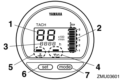
1. Drehzahlmesser 2. Trimmanzeige 3. Betriebsstundenzähler 4. Warnleuchte niedriger Öldruck 5. Überhitzungs-Warnleuchte 6. Einstelltaste 7. Modustaste
