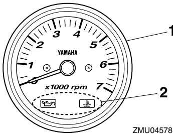
1. Drehzahlmesser 2. Warnungsanzeige(n)
