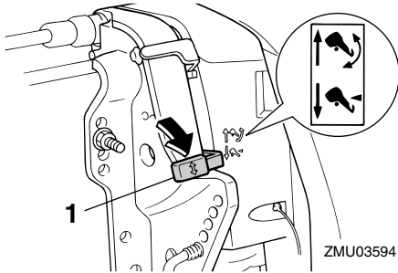
1. Kipperrhebel
