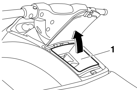
1 Porta-luvas
