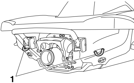
1 Hecköse
